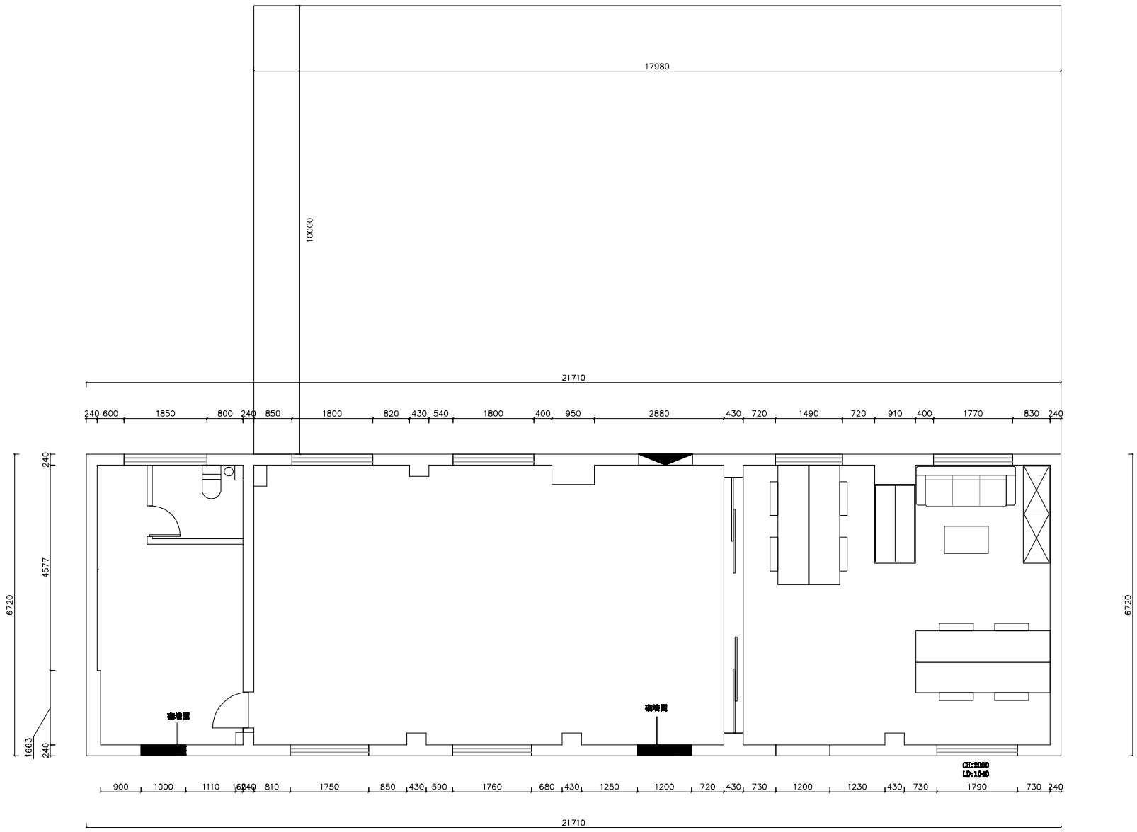
平面图
