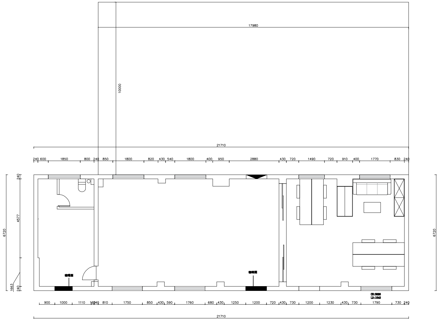
平面图
